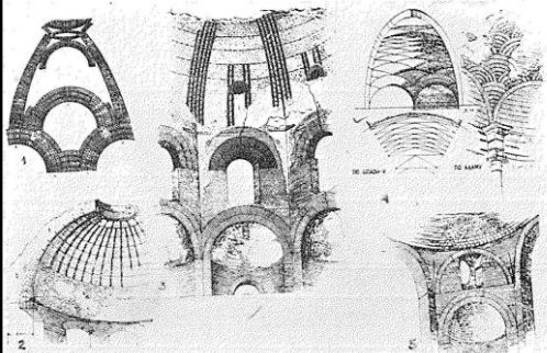
Sl. 247. Konstrukcije rimskih kupola. 1 — Panteon; 2 — Hram u Tivoliju; 3 — Hram Minerve Medike; 4 — Dioklecijanov mauzolej u Splitu; 5 — Karakaline terme u Rimu
