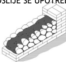
OPUS INCERTUM
