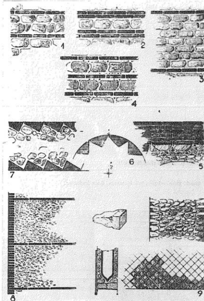
Sl. 240. Rimski vezovi zidanja — opusi. 1, 2, 3, 4, 5 — opus mixtum, (miješani zid — kamen i opeka); 6, 7, 8 — opus cementicum (emplekton) — betonski liv sa kamenom oblogom; 9 — opus reticulatum (mrežasti vez) — liv sa oblogom od malih kamenih kocki.
